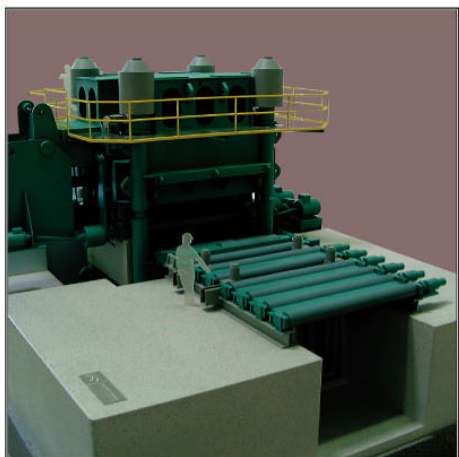
Planeuse - Ech : 1/15 1300 x 800mm
