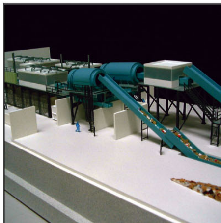
Centre de tri - Ech : 1/100 1100 x 350mm
